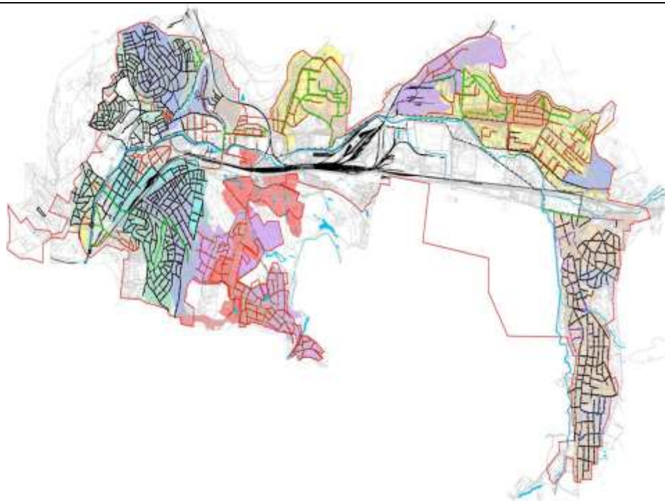
Канализационна схема на град Радомир:
